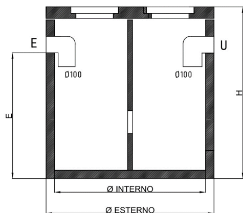
SEZIONE VERTICALE
